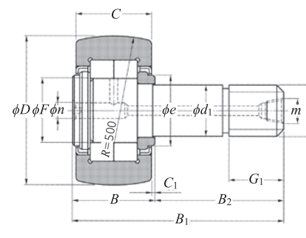
NUKR type ( D \geq 100 mm)
