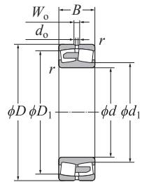
Cylindrical bore [Type EM (large size)]
