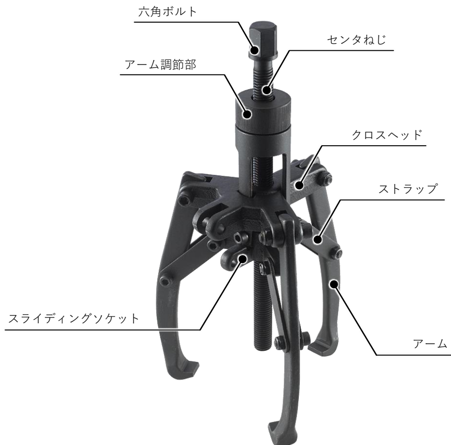
図 4.1 引抜き治具(3品番共通)
