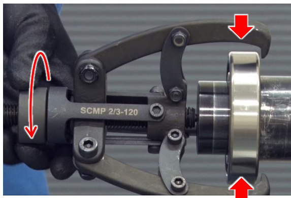
図 5.6 引抜き治具の固定(1)
