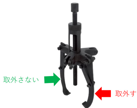
図 5.16 2本アームから3本アームへの変更
