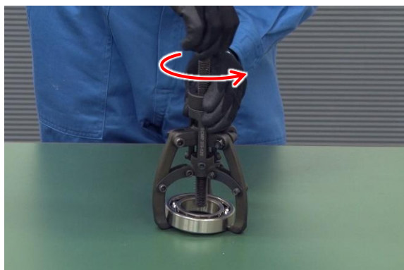
図 5.9 軸受の取出し
