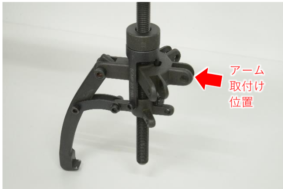
図 5.14 アーム取付け位置
