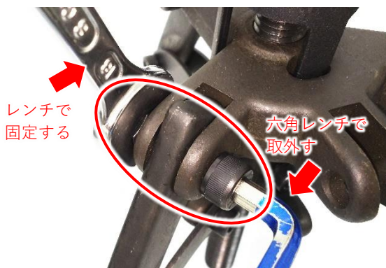
図 5.13 アーム取外し位置
