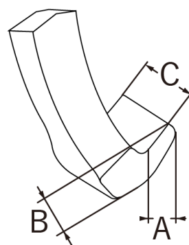
図 8.2 爪寸法
