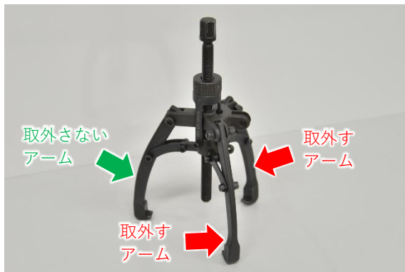
図 5.11 取外すアーム
