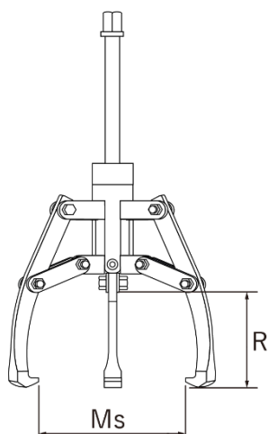
図 8.1 対応径 M_s 及び最大長さ R の寸法線
