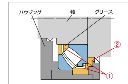
図2 横軸でのグリース封入状態
