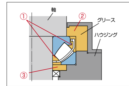
図1 立軸でのグリース封入状態
